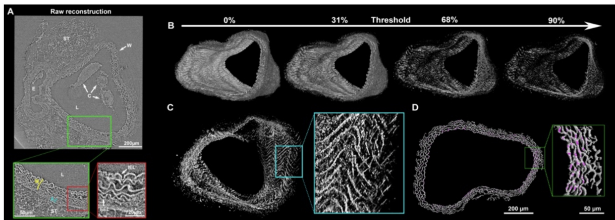
Figure 1: Image \mu CT acquise sur synchrotron (coupe 2D, à gauche) et structures extraites / visualisées à partir de cette image (visualisation 3D à droite).
